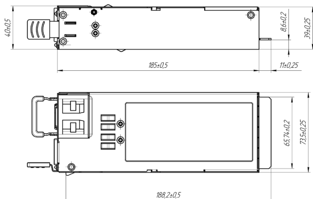
Габаритный чертеж КАНВ800C12, габариты в мм
