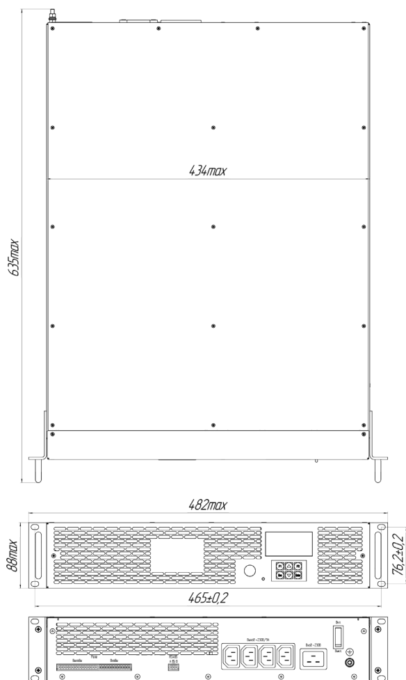
Габаритный чертеж ИБП «Поток», габариты в мм.
