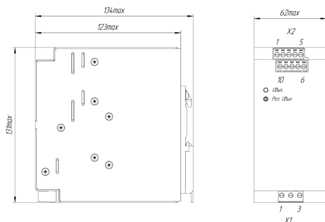
Габаритный чертеж КАН-Д480C24, габариты в мм
